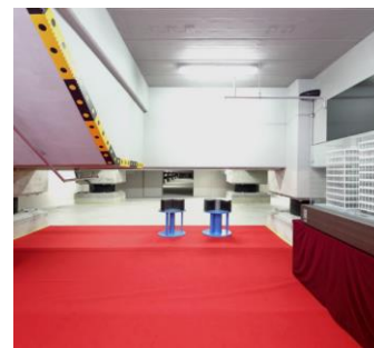
면진시설 : 바닥 및 벽체의 면진 구조(특허출원)
